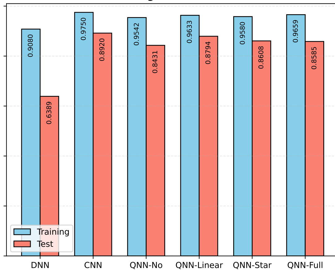
OrganAMNIST
