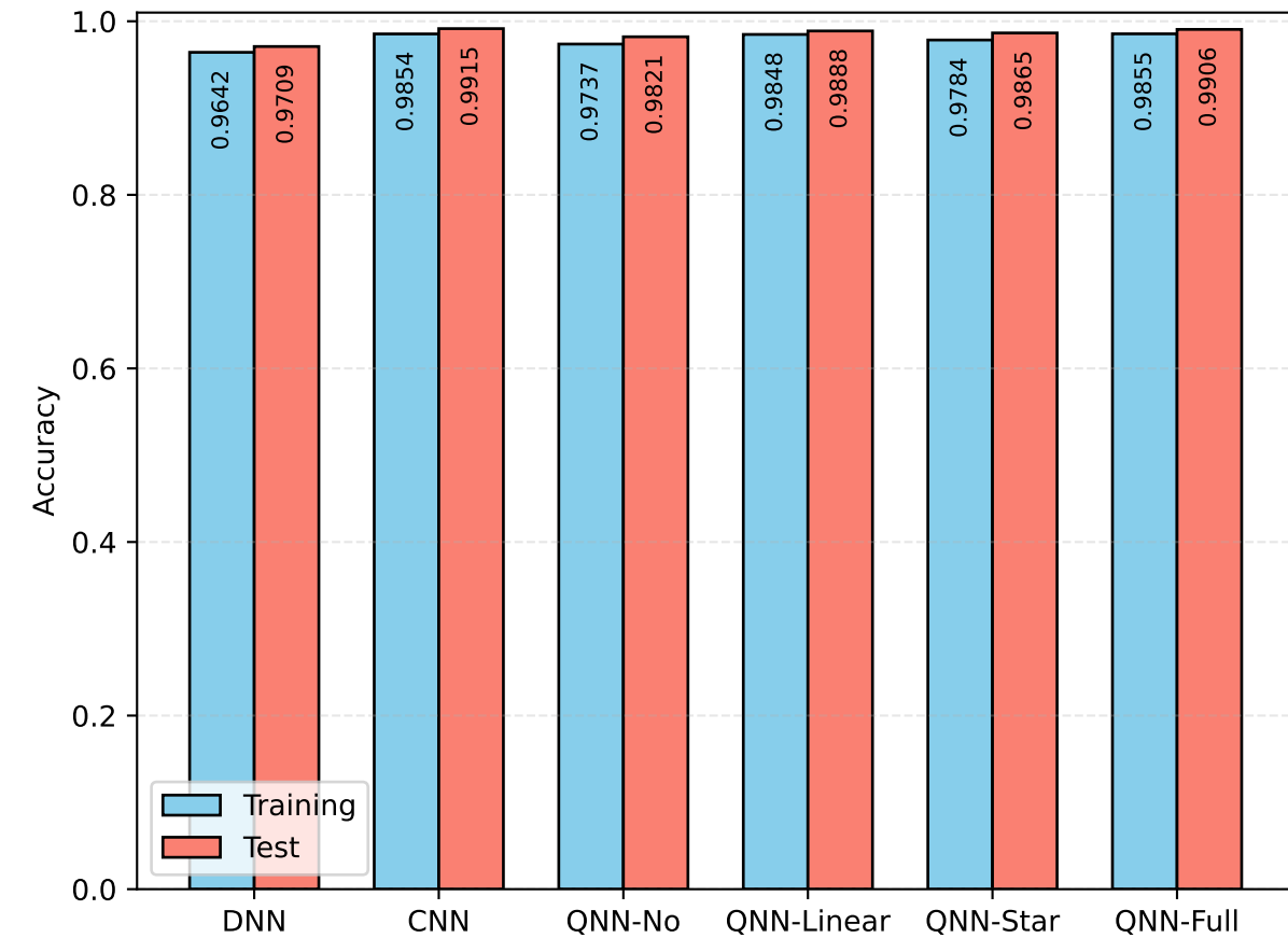
MNIST
